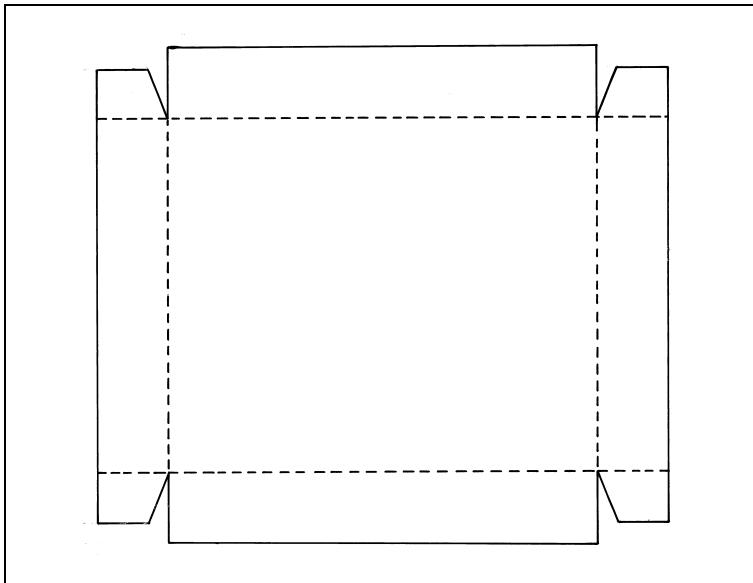
Abb. 8-5: Geritzte Schachtel
