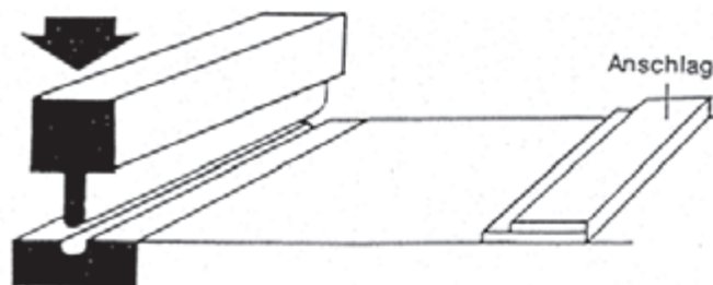
Schema eines Rillgerätes
